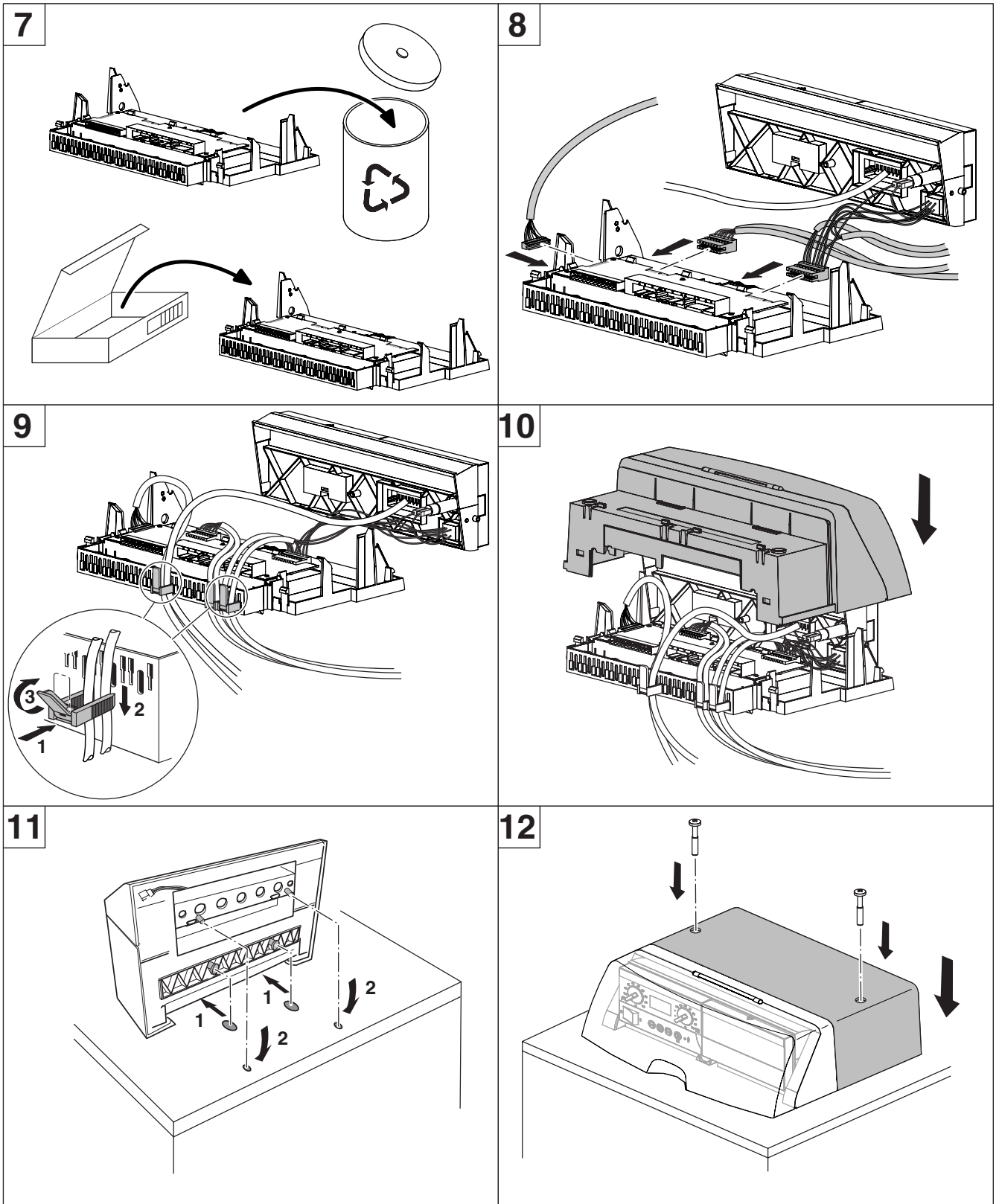
Bild 2: Austausch HC10
