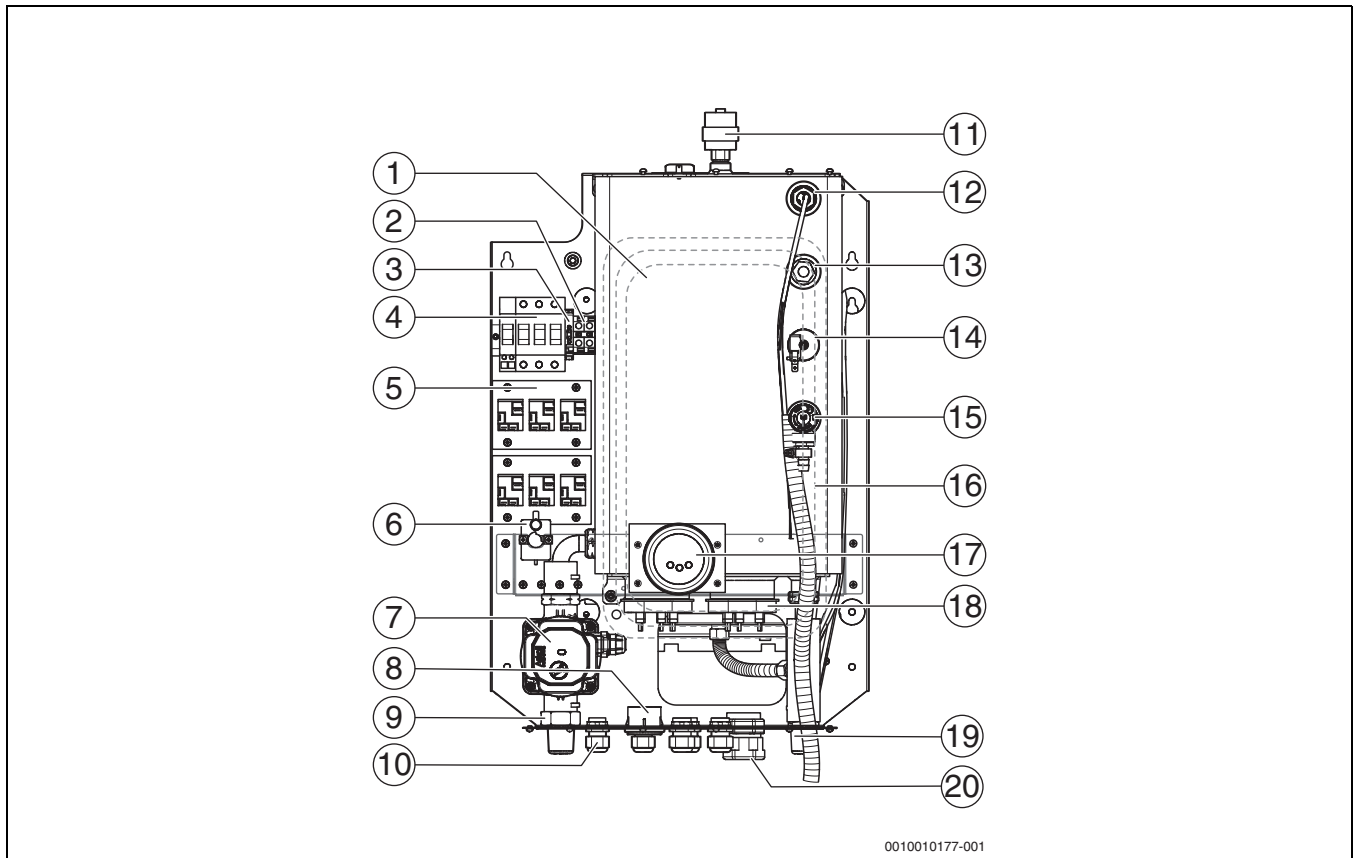
Bild 2 Funktionselemente des Heizgerätes Logamax E156 15-24 kW
