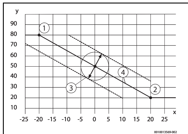
Bild 4 Außentemperaturgeführte Heizkurve
