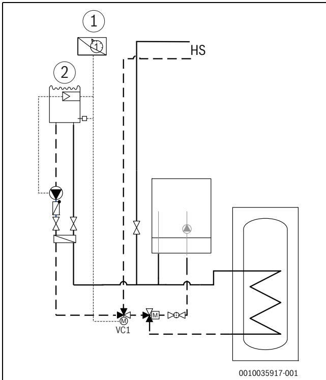
Bild 27 Beispieldarstellung für Pool-Installation
