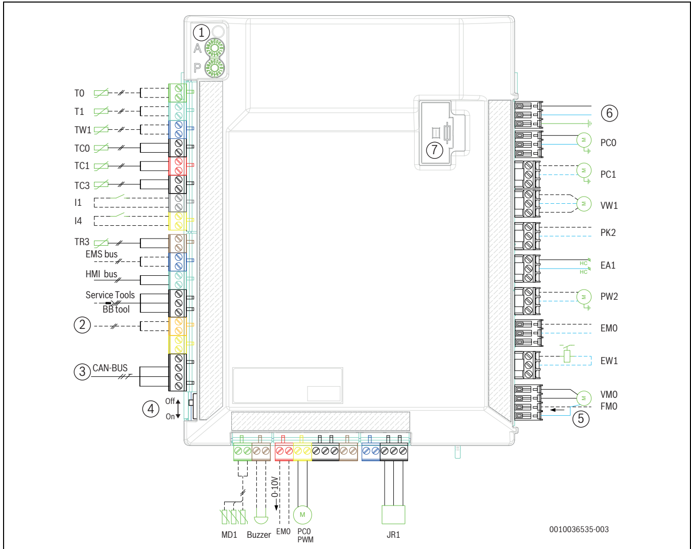
Bild 37 Installationsleiterplatte der Inneneinheit
