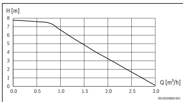
Bild 29 Leistungskurve der Primärumwälzpumpe (PCO)
