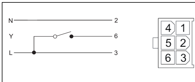
Bild 23 Molex-Stecker
