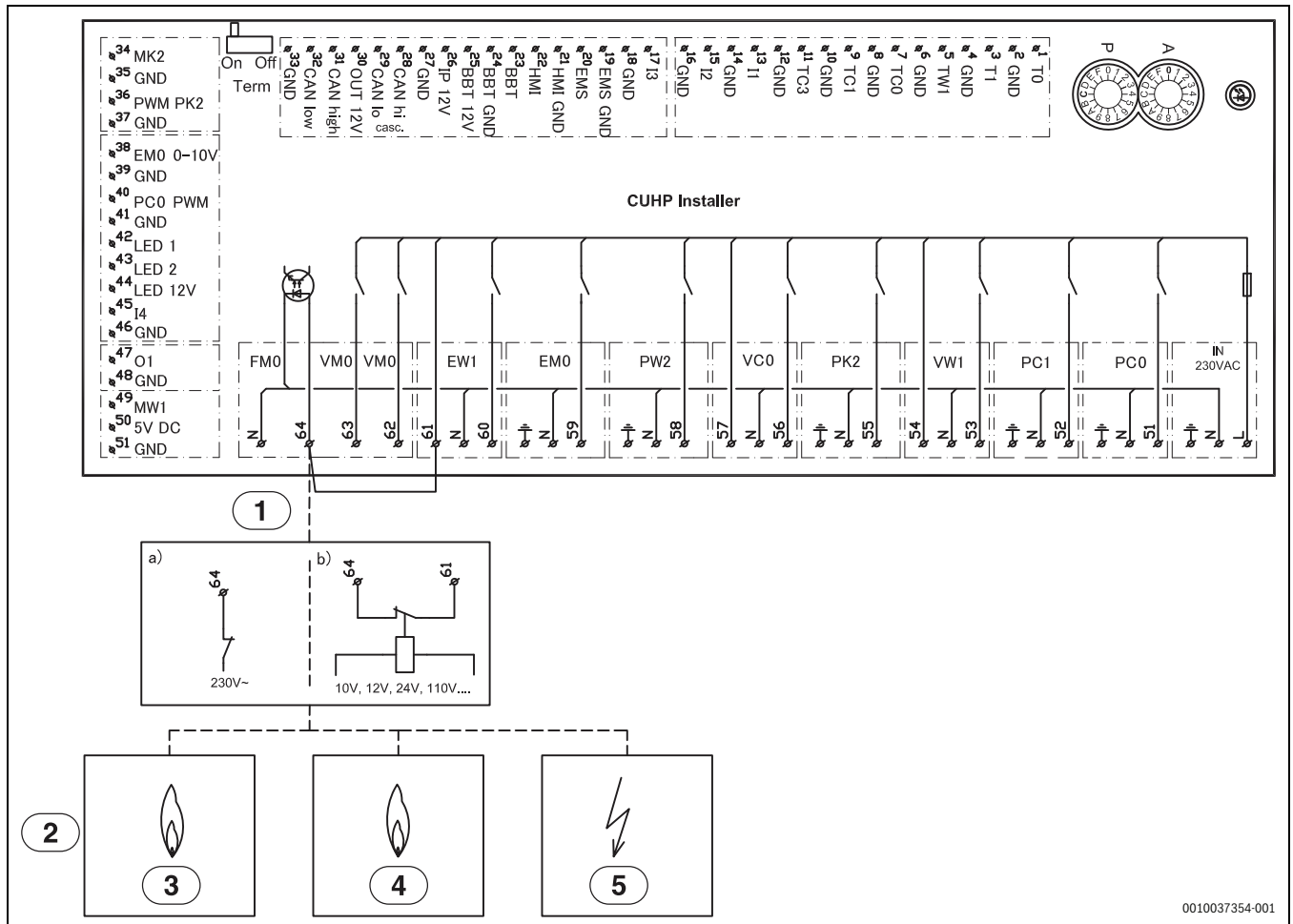
Bild 15 Schaltschema der Installationsleiterplatte, Alarm für externen Zuheizer
