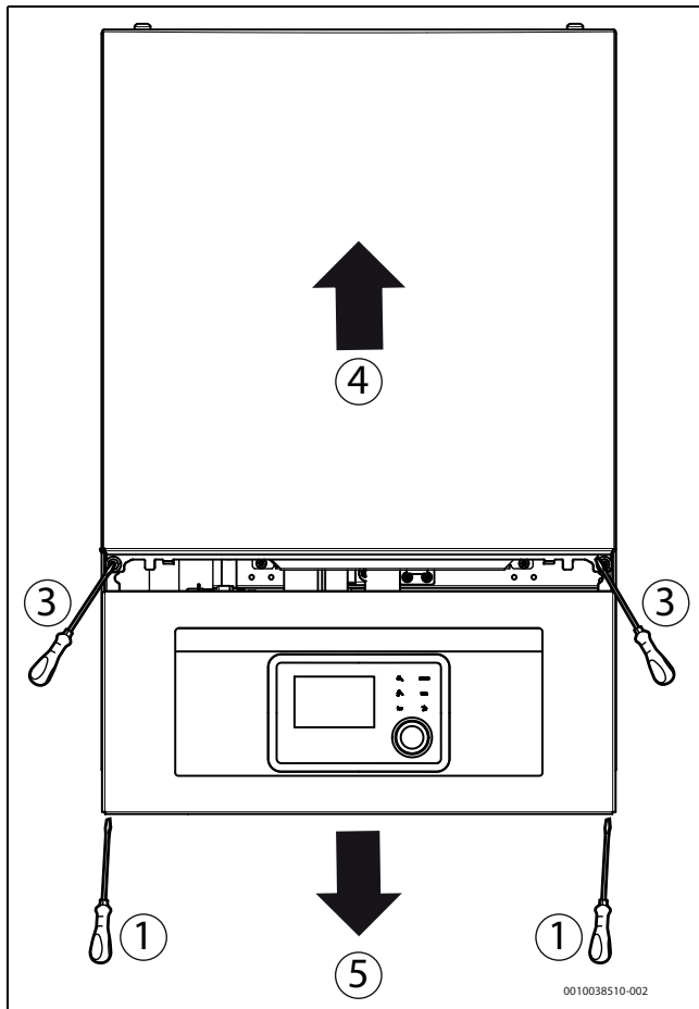
Bild 6 Frontverkleidung abnehmen
