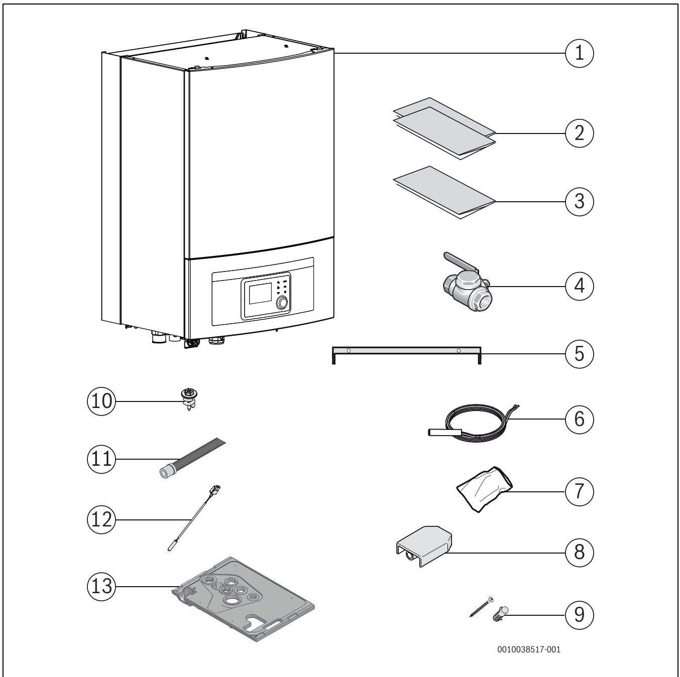
Bild 2 Lieferumfang
