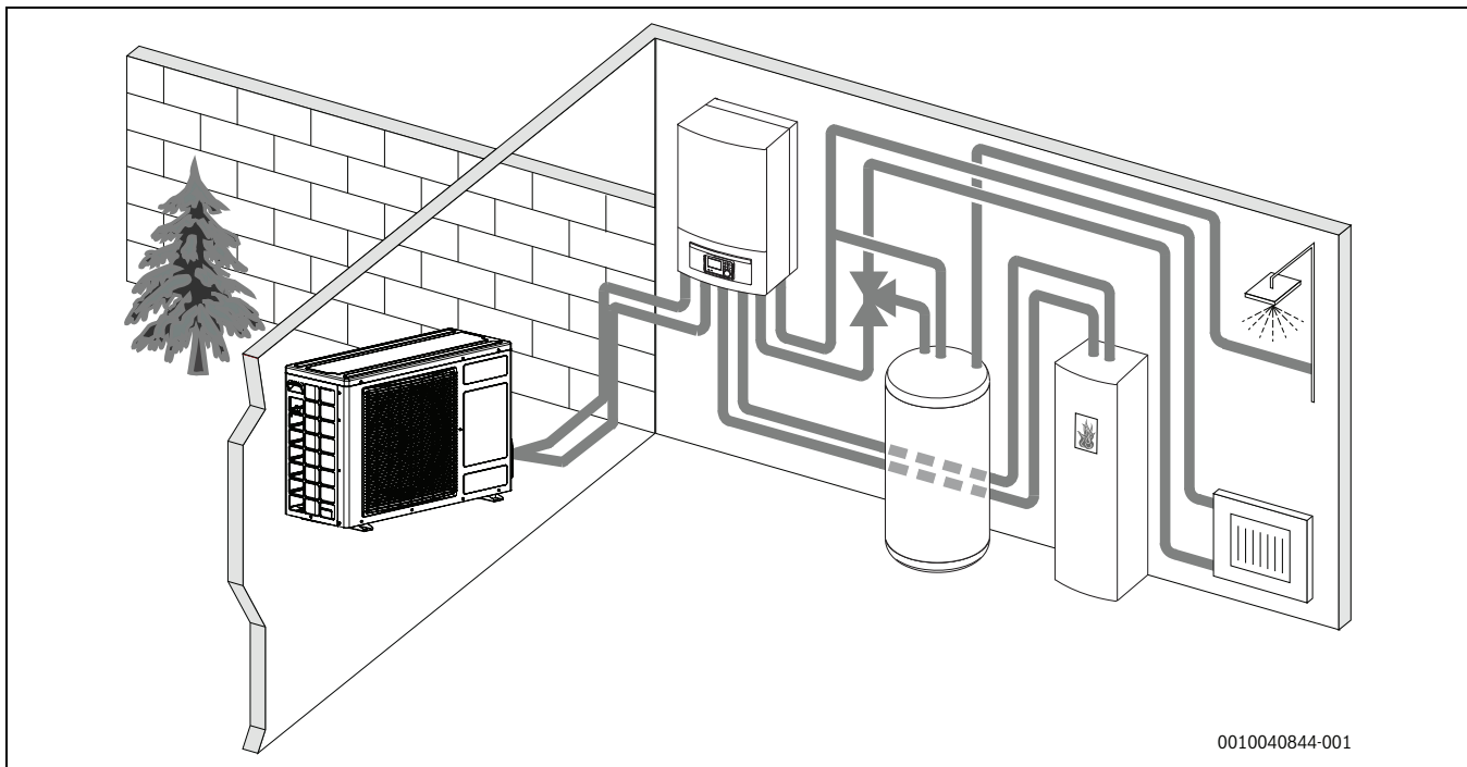
Bild 2 Wärmepumpe als Außeneinheit, Inneneinheit WLW166i B ohne elektrischen Zuheizer, externer Warmwasserspeicher und externer Zuheizer
