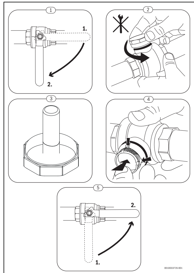
Bild 6 Siebreinigung
