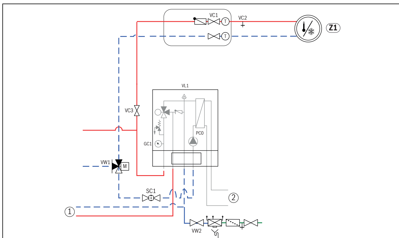
Bild 9 Inneneinheit mit externem Zuheizung und Heizsystem
