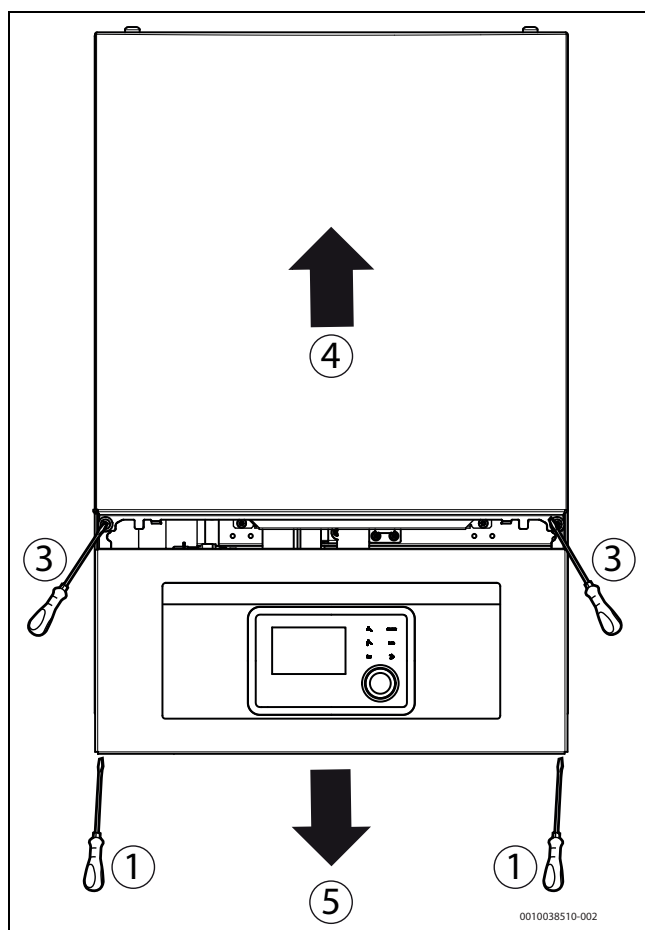
Bild 6 Frontverkleidung abnehmen
