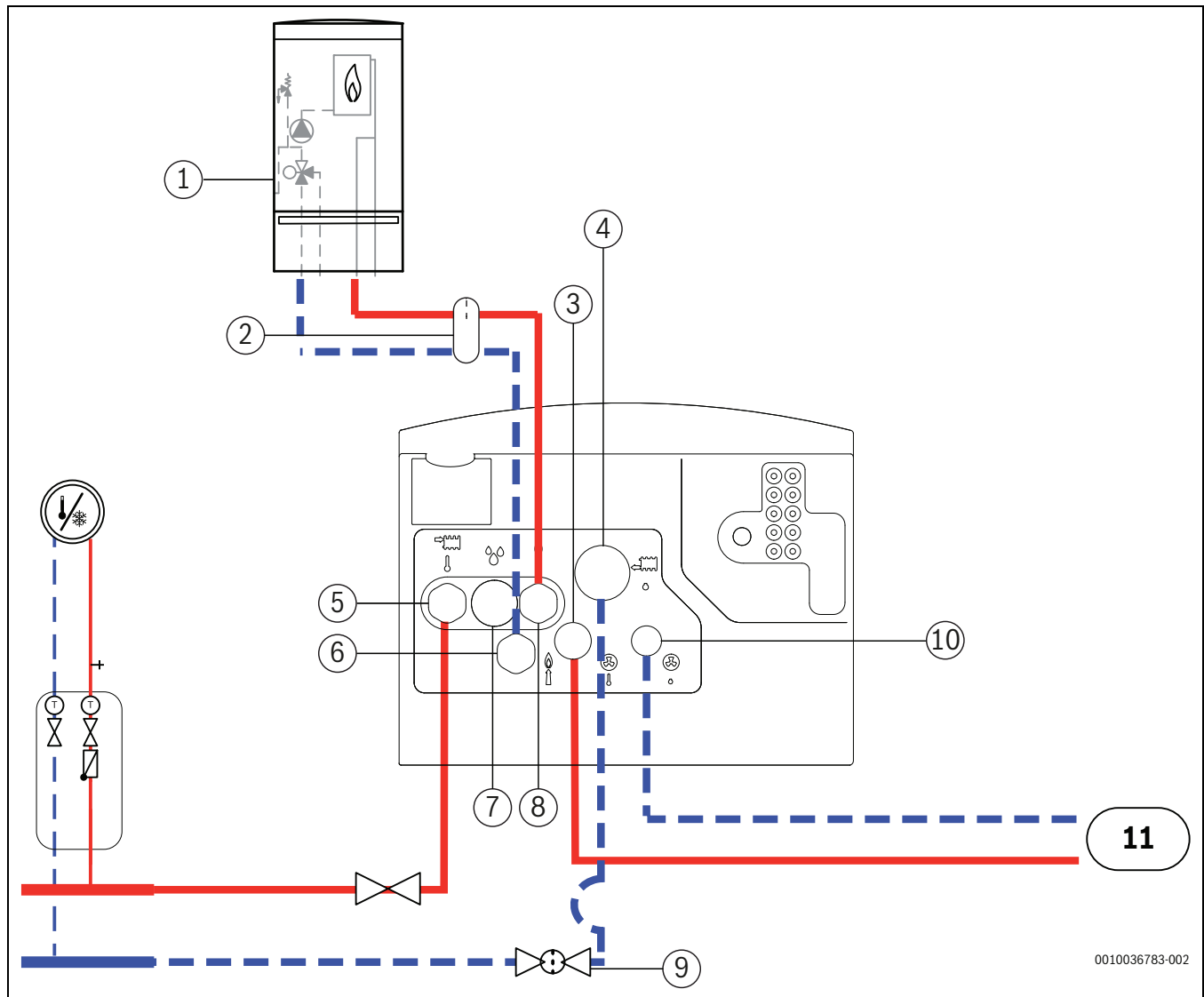
Bild 8 Anschluss der Inneneinheit mit Mischer für externen Zuheizter an die Heizungsanlage und den Zuheizter
