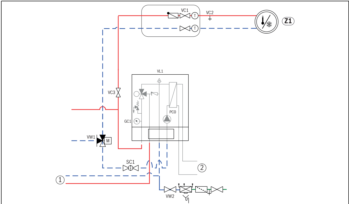
Bild 18 Inneneinheit mit externem Zuheizer und Heizsystem
