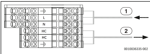
Bild 16 Anschlussklemmen für elektrischen Anschluss
