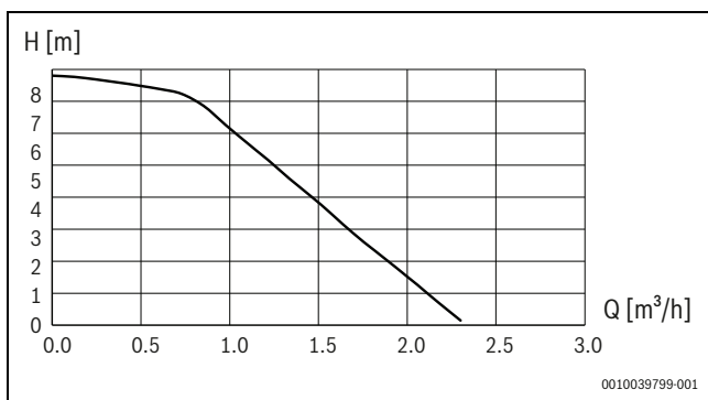
Bild 29 Leistungskurve der Primärsumwälzpumpe (PC0)
