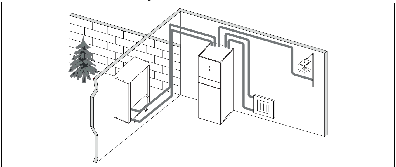
Bild 3 Wärmepumpe WLW196i.2 AR/IR, Inneneinheit IDU-..iT / IDU-..iTS mit integriertem Warmwasserspeicher und elektrischem Zuheizter
