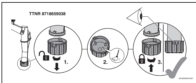
Bild 90 Schmutzfänger reinigen
