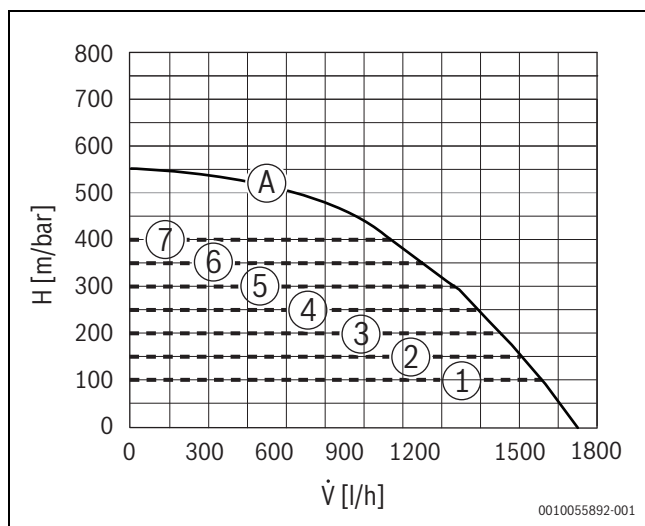
Bild 99 Pumpenkennfelder und Pumpenkennlinien
