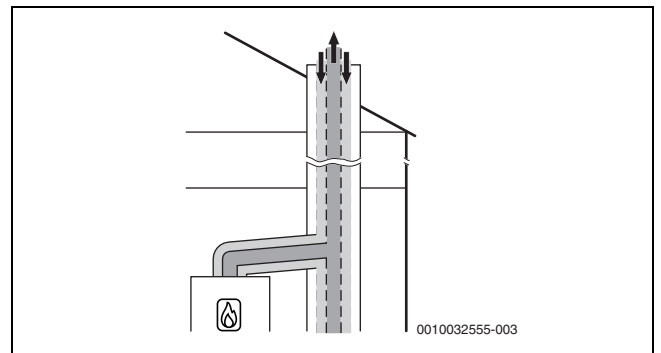
Bild 18 Konzentrische Luft-Abgas-Führung nach C 43x im Aufstellraum
