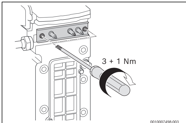
Bild 78 Elektroden-Set montieren
