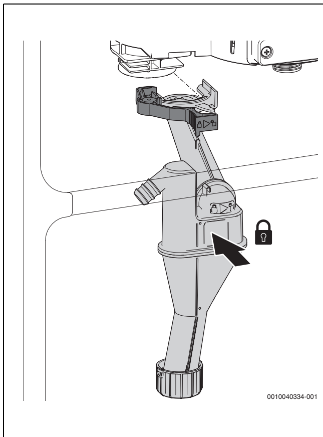
Bild 93 Kondensatsiphon einsetzen
