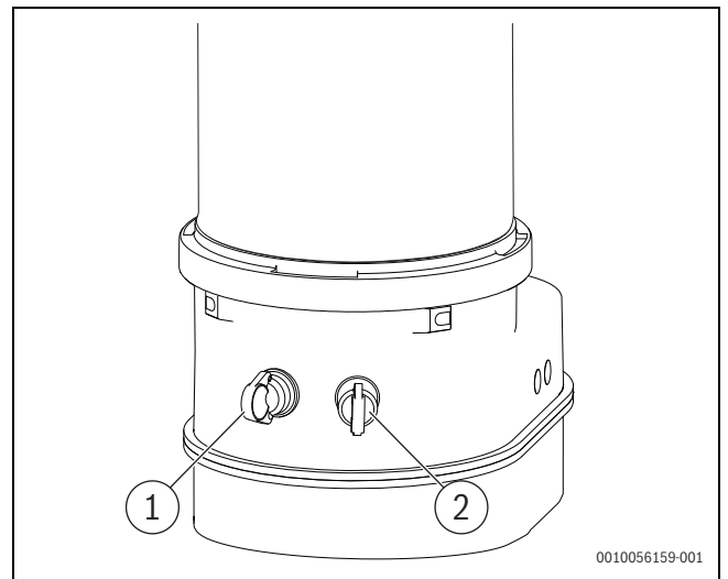
Bild 77 Abgasmessstutzen und Verbrennungsluft-Messstutzen
