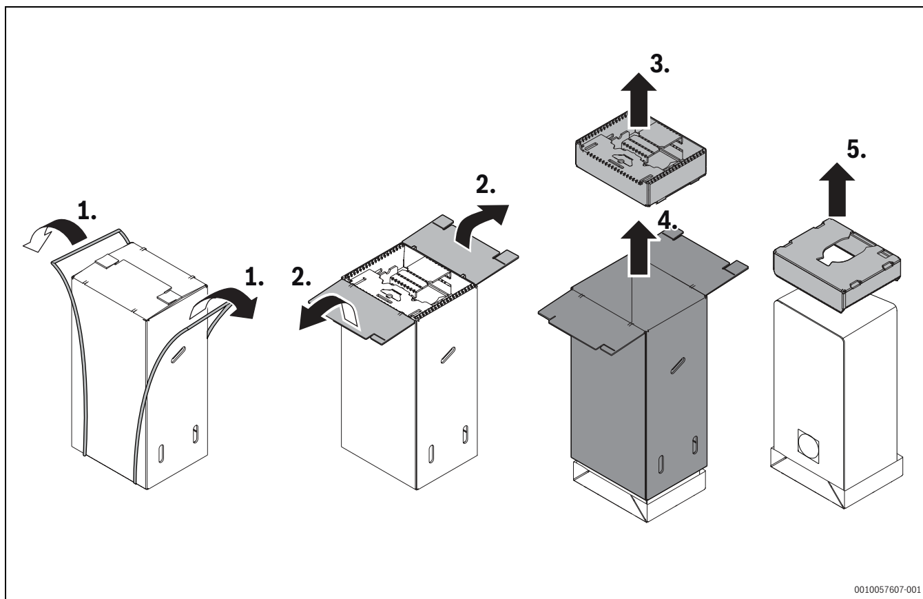
Bild 38 Auspackanweisung
