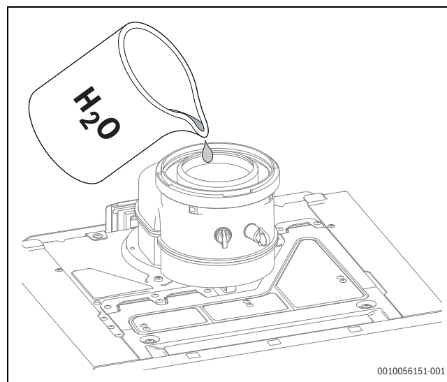
Bild 59 Kondensatsiphon mit Wasser füllen
