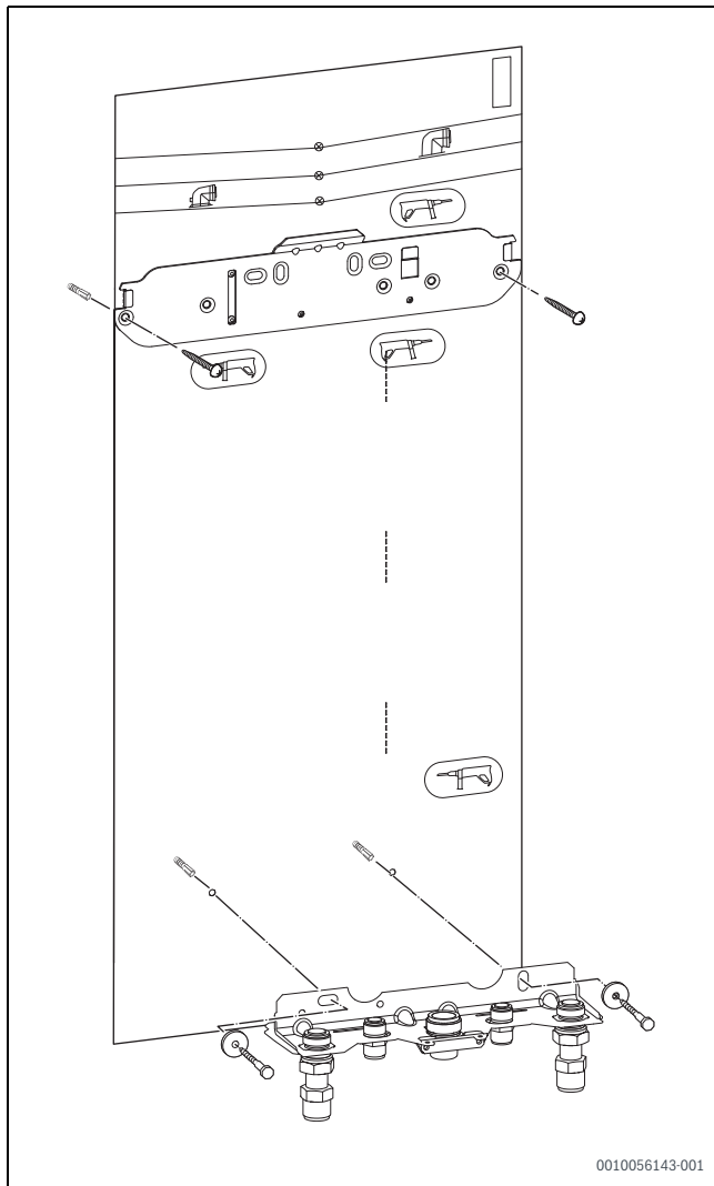
Bild 39 Haltebühle und Montageanschlussplatte montieren
