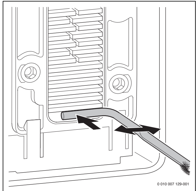
Bild 88 Kondensatwanne reinigen
