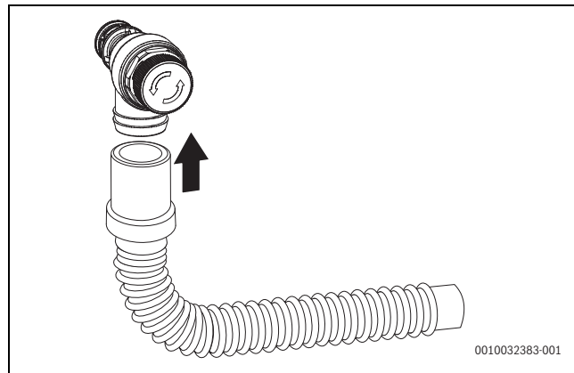
Bild 55 Schlauch am Sicherheitsventil (Heizung) montieren
