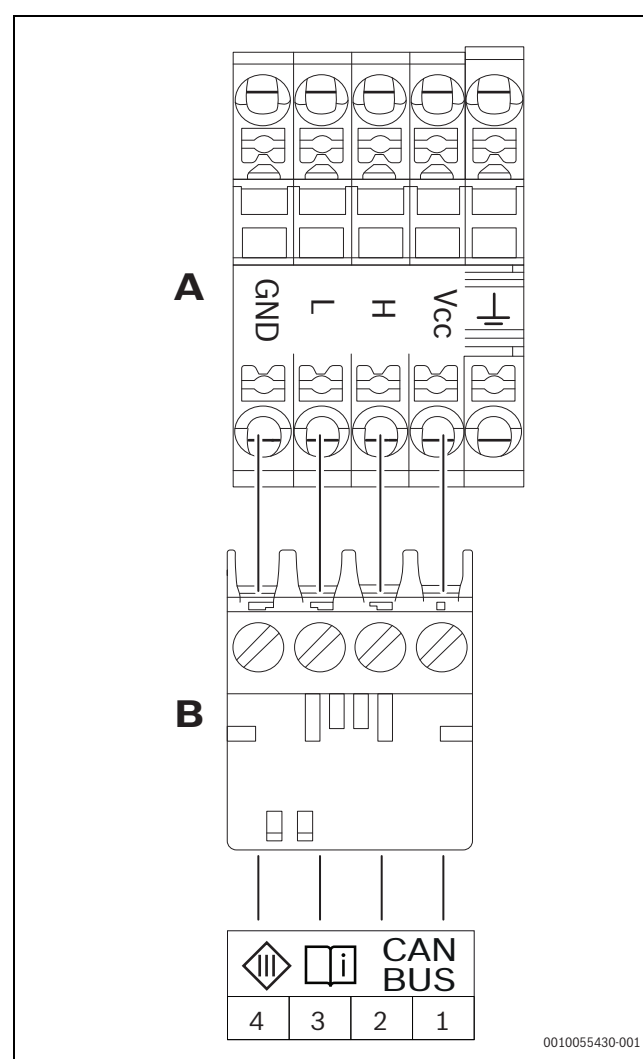
Bild 53 CAN-BUS Außeneinheit - Heizgerät
