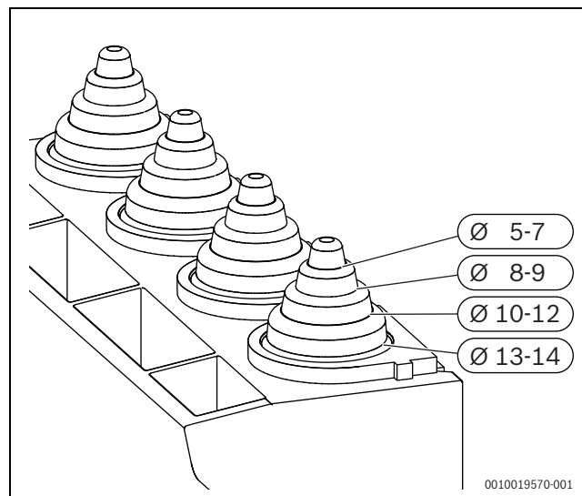
Bild 63 Zugentlastung an Kabeldurchmesser anpassen
