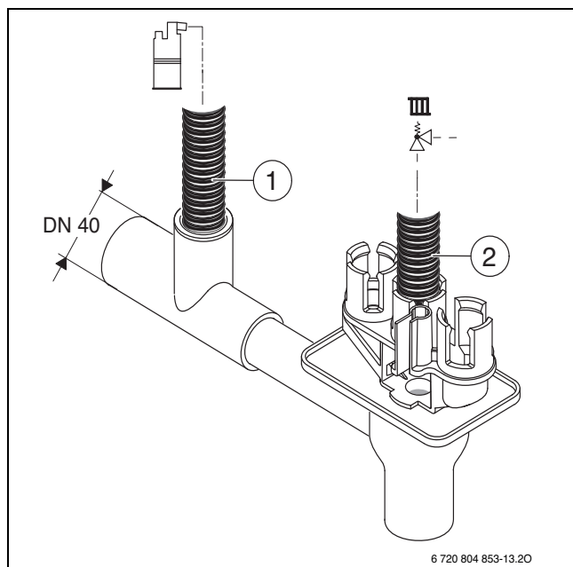
Bild 57 Kondensatschlauch und Schlauch vom Sicherheitsventil am Siphon montieren
