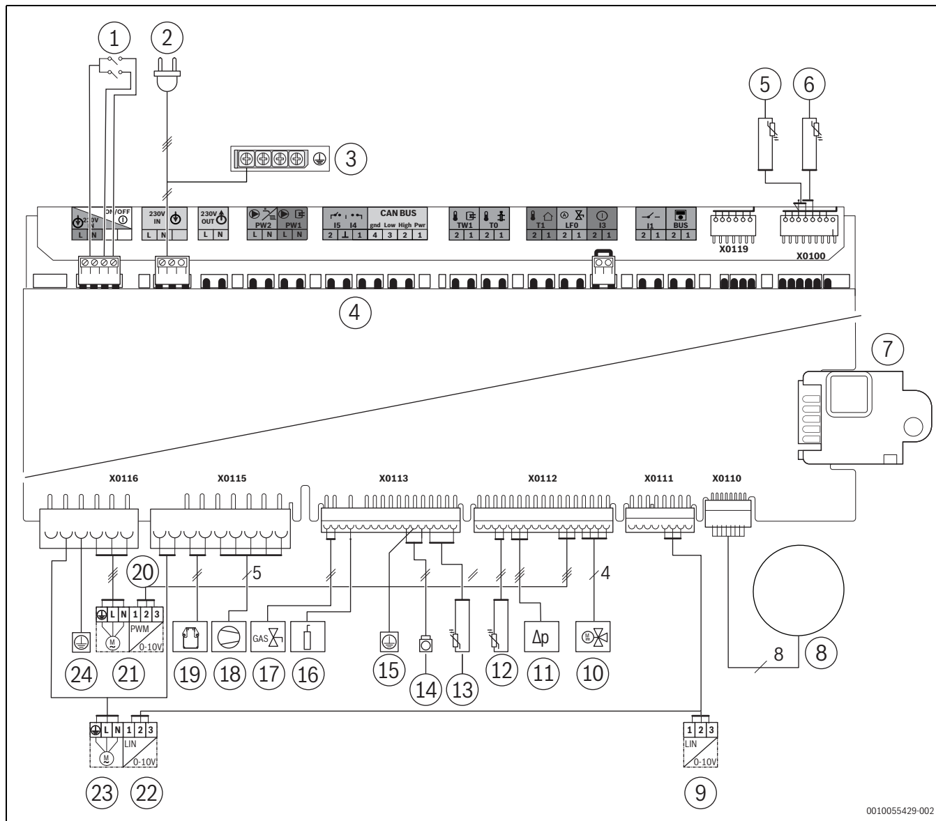
Bild 100 Elektrische Verdrahtung
