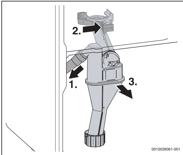
Bild 89 Kondensatsiphon ausbauen
