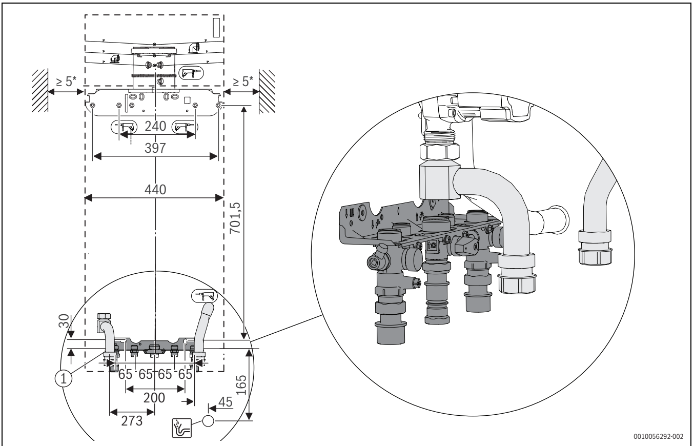
Bild 3 Vorderansicht (mm)
