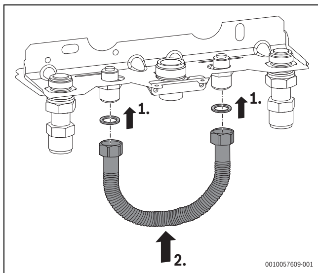
Bild 51 Warmwasser-Bypassleitung (7107800) installieren
