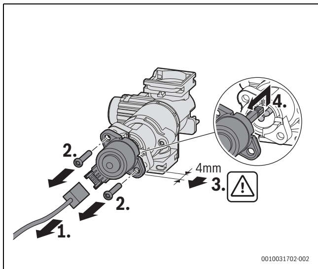
Bild 97 Motor am 3-Wege-Ventil ausbauen (Variante mit Schrauben)
