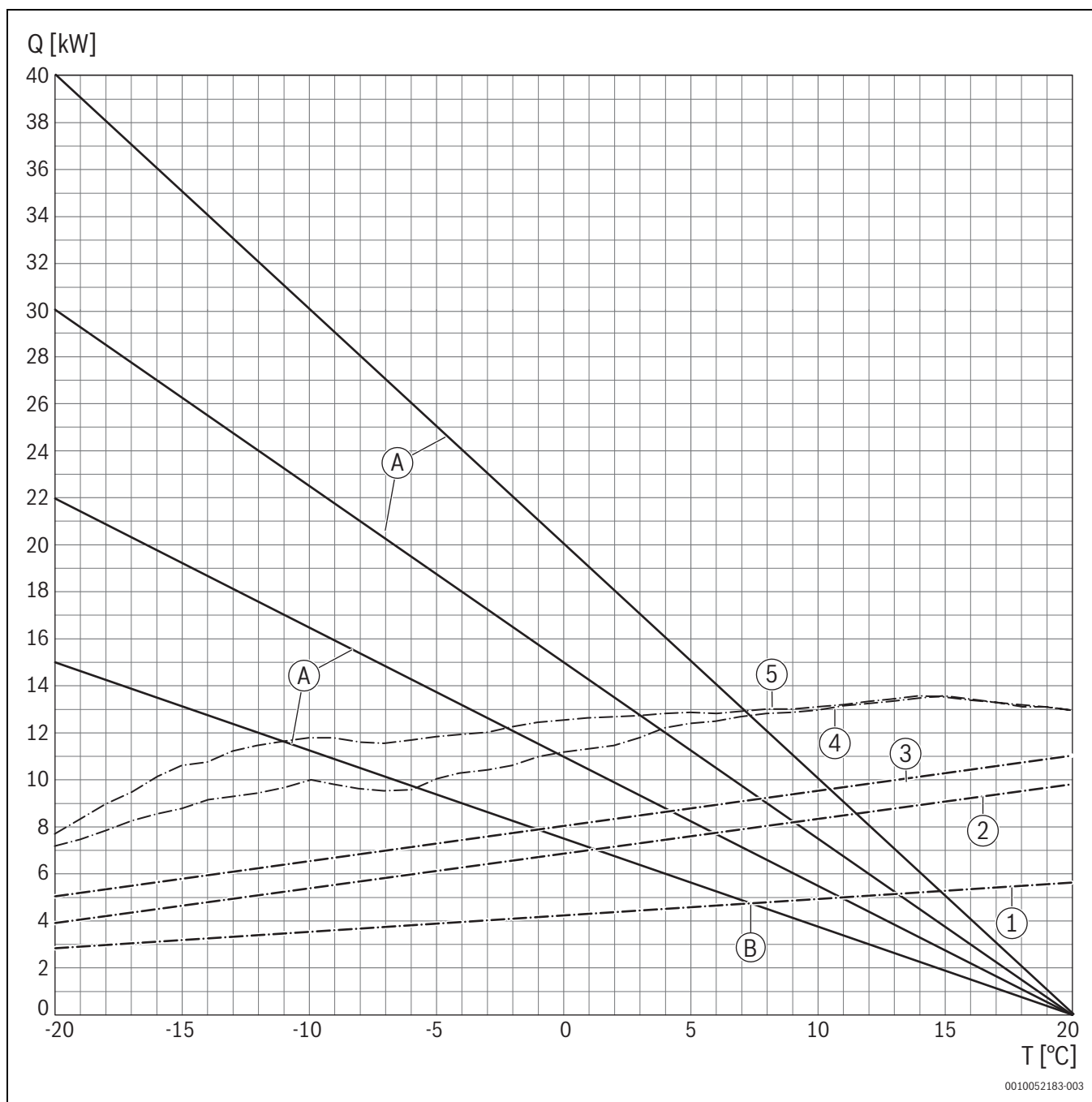
Bild 69 Diagramm für Tab. 92 zur Bestimmung der Bivalenztemperaturen bei einer Vorlauftemperatur von 35 °C
