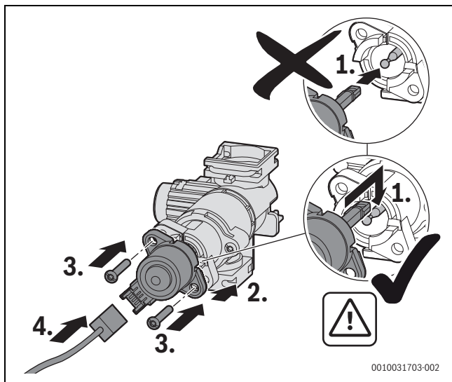
Bild 98 Motor im 3-Wege-Ventil installieren (Variante mit Schrauben)
