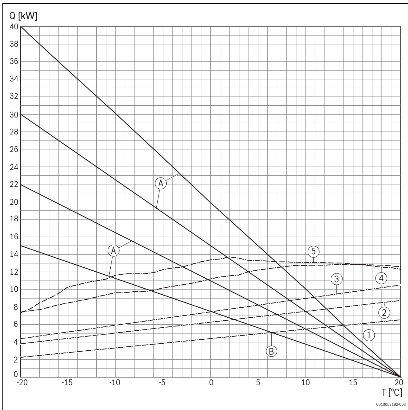
Bild 70 Diagramm für Tab. 93 zur Bestimmung der Bivalenztemperaturen bei einer Vorlauftemperatur von 45 °C
