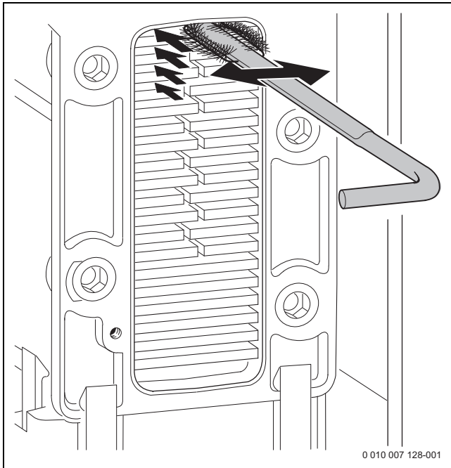
Bild 86 Wärmeblock mit Bürste reinigen
