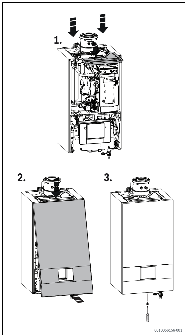
Bild 67 Verkleidung montieren
