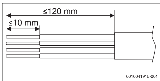
Bild 54 Abisolierung CAN-BUS
