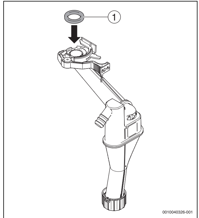
Bild 91 Neue Dichtung am Kondensatsiphon einsetzen
