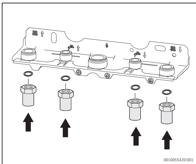
Bild 40 Rohre mit Dichtungen an Montageanschlussplatte montieren
