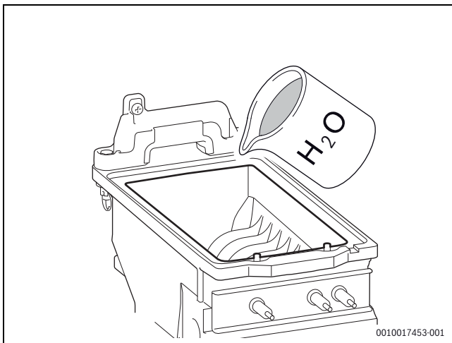
Bild 87 Wärmeblock spülen
