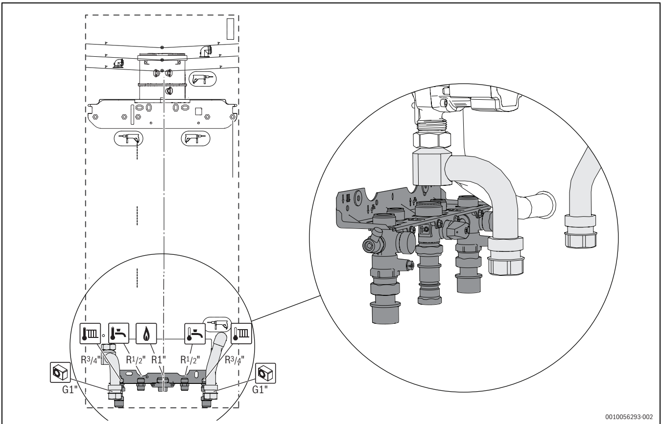
Bild 4 Vorderansicht (Anschlüsse)
