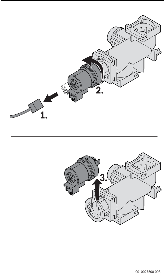
Bild 95 Motor vom 3-Wege-Ventil lösen (Variante ohne Schrauben)
