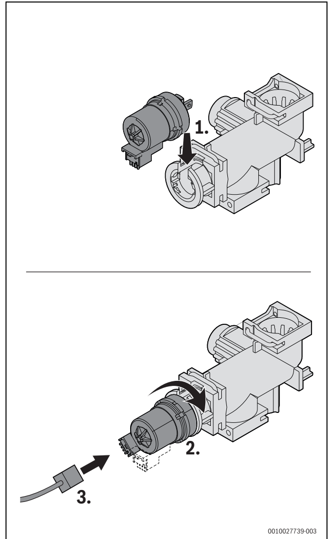
Bild 96 Motor im 3-Wege-Ventil installieren (Variante ohne Schrauben)
