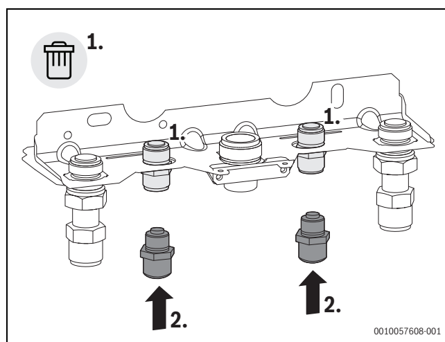
Bild 50 Anschlussadapter (7738112656) ersetzen
