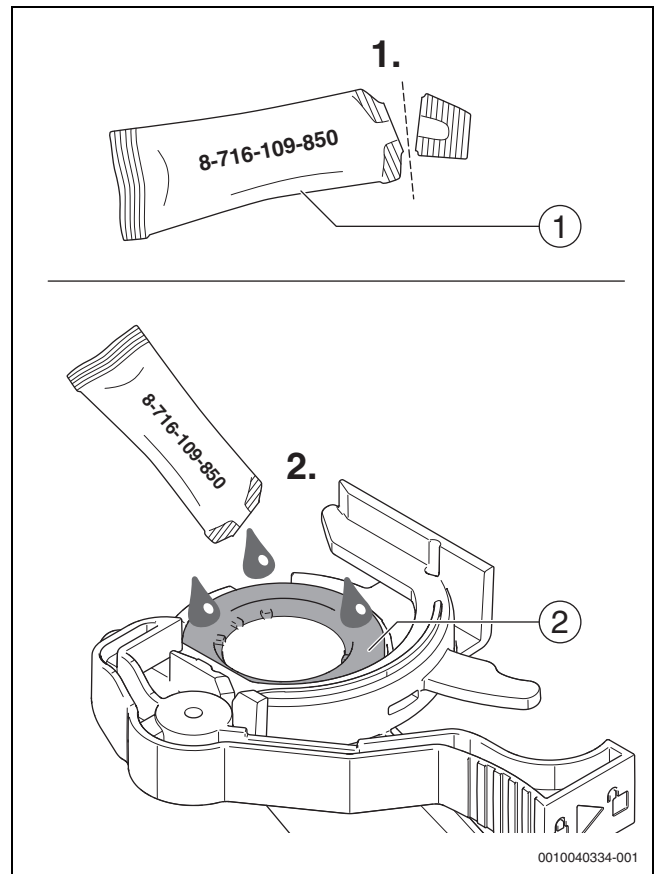
Bild 92 Dichtung fetten
