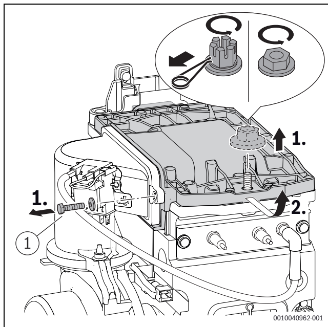
Bild 80 Brennerdeckel ausbauen
