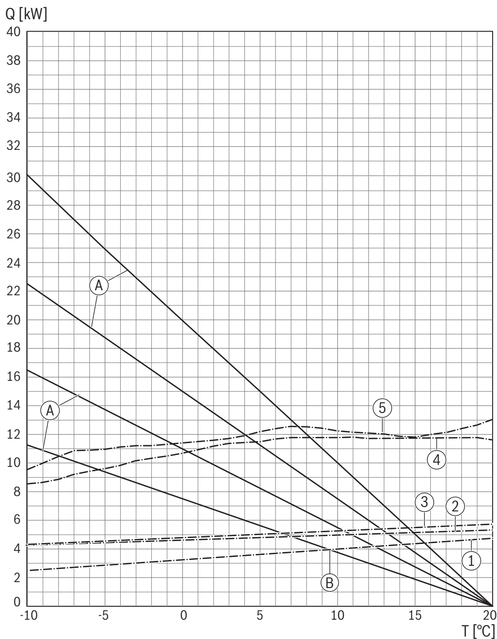
Bild 72 Diagramm für Tabelle 95 zur Bestimmung der Bivalenztemperaturen bei einer Vorlauftemperatur von 65 °C
