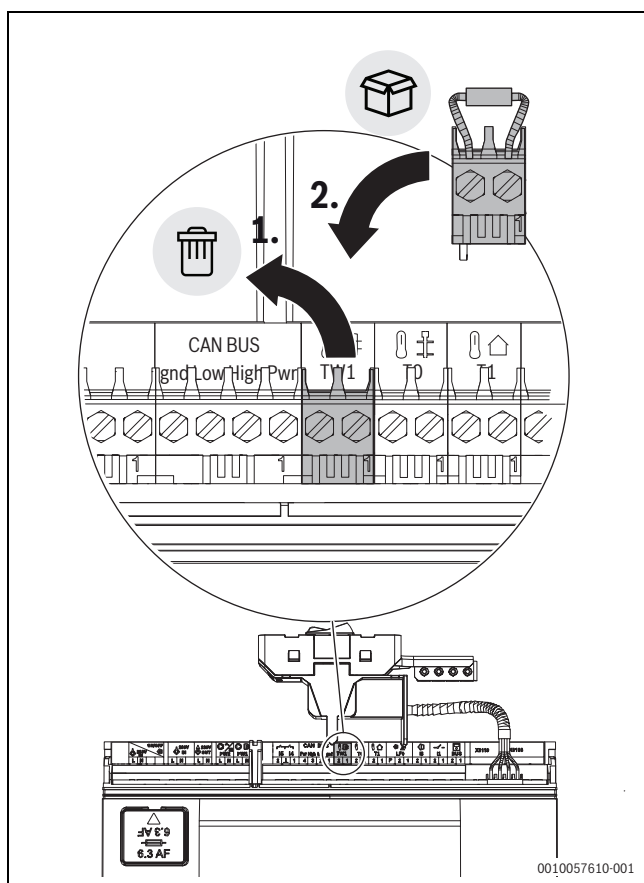
Bild 52 Steckverbinder mit Widerstand (7738114115) installieren
