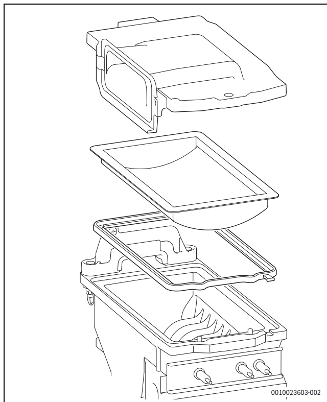
Bild 81 Brenner
