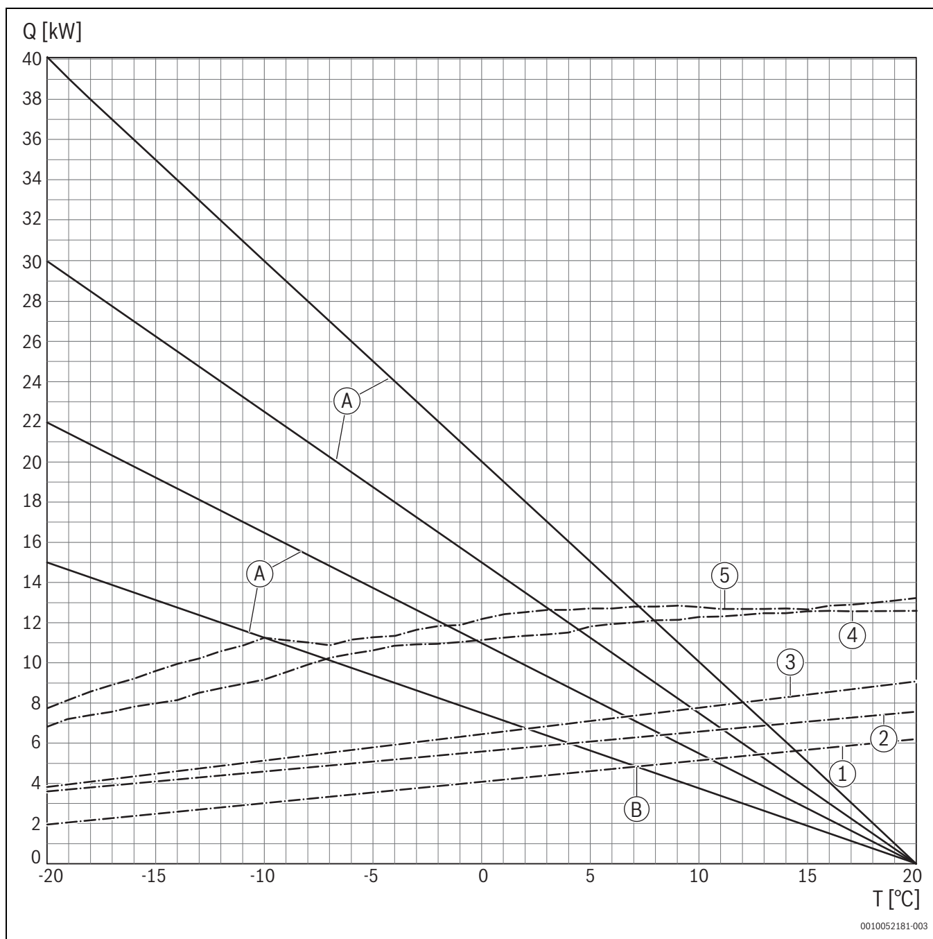
Bild 71 Diagramm für Tab. 94 zur Bestimmung der Bivalenztemperaturen bei einer Vorlauftemperatur von 55 °C
